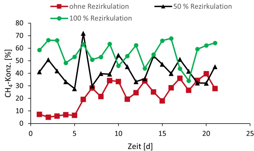
Abbildung 1: Methangehalt im Biogas bei unterschiedlichen Dünnschlammrezirkulationsmengen in der methanogenen Prozessstufe (© TU Berlin)
