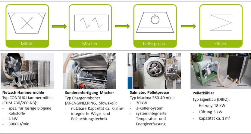
Abbildung 2 Pelletherstellungsprozess am DBFZ (©DBFZ: 2018)
