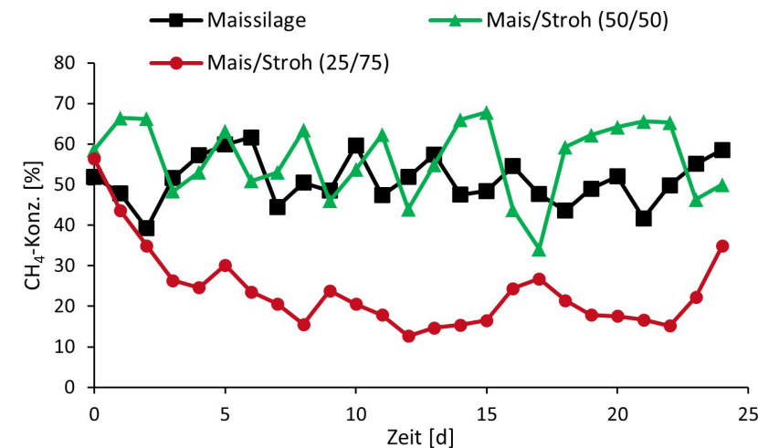
Abbildung 2: Methangehalt im Biogas bei unterschiedlicher Substratzusammensetzung (© TU Berlin)
