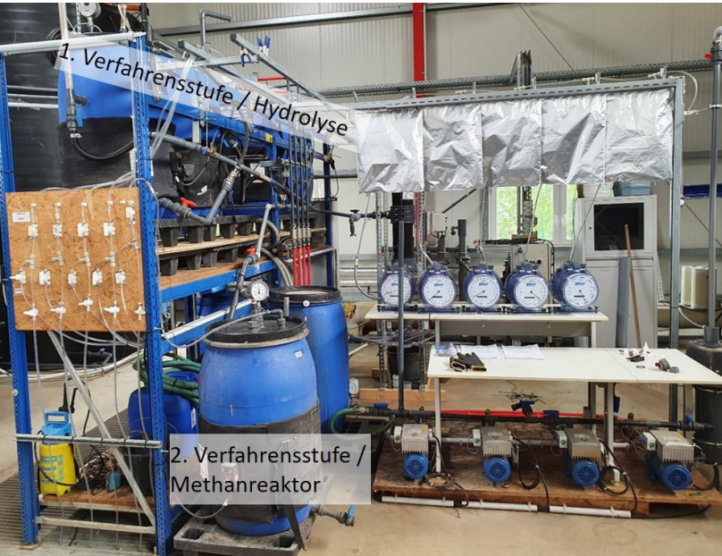
Abbildung 8: Gesamtansicht Demonstrationsanlage nach Umbau und Einbindung des AEV-Mehrphasenabscheiders (© GICON)
