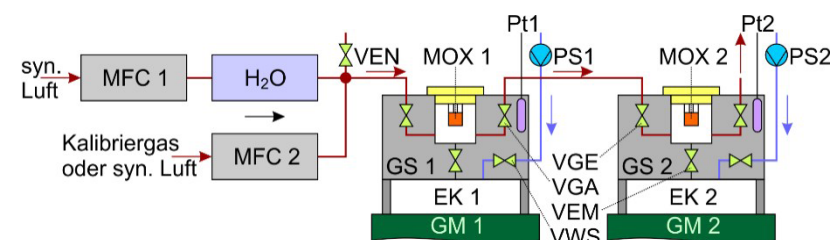
Abbildung 3: Fluidische Verbindungen für die Ansteuerung der Gelöstgassensoren GS1/2 mit integrierten Metalloxid-Gassensoren MOX1/2, MFC= Massendurchflussregler, H 2 O=Gasbefuchtung, EK= Extraktionskammer, GM= Gärmedium, Vxx= Ventile für Gaseinlass, Gasauslass, Messgasdiffusion, Wasserspülung und Druckentlastung. (© KSI Meinsberg)
