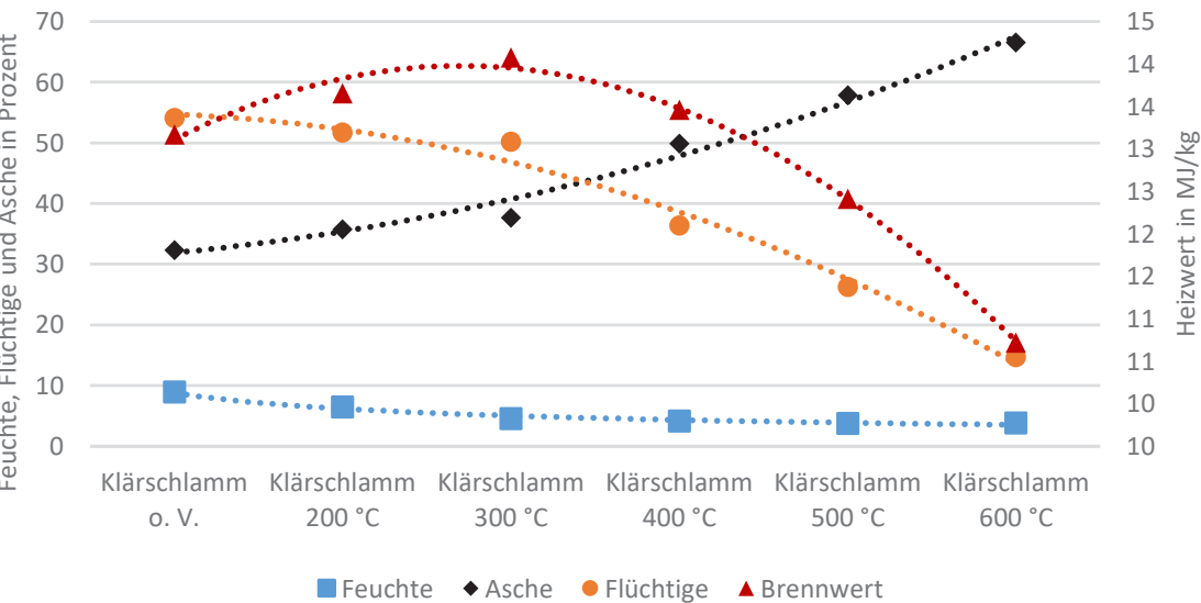
Abbildung 1: Ergebnisse der Brennstoffanalyse von Klärschlamm bei unterschiedlichen Vorbehandlungstemperaturen (© TU München)
