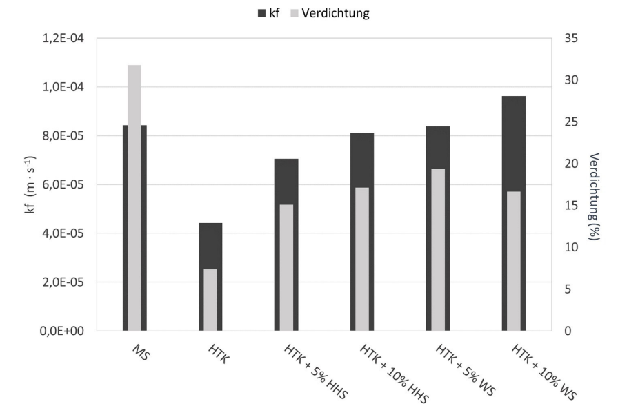
Abbildung 5: kf-Wert und Verdichtung der unter-suchten HTK Proben mit unterschied-lichen Anteilen an Strukturmaterial gemessen bei einer Auflast von 3 bar (MS, Maissilage; HHS, Holzhackschnitzel; WS, Weizenstroh) (© DBFZ)
