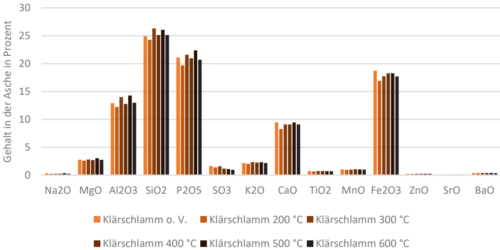
Abbildung 2: Zusammensetzung der Asche von Klärschlamm bei unterschiedlichen Vorbehandlungstemperaturen (© TU München)
