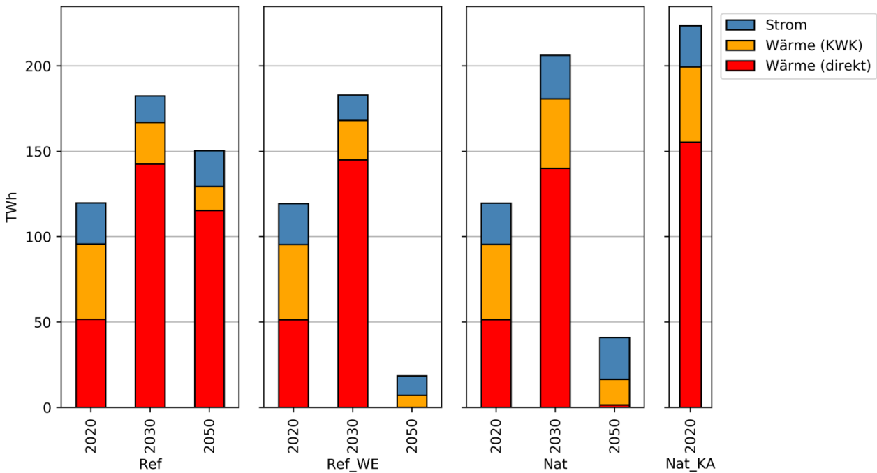
Abbildung 4-2: Strom- und Wärmeerzeugung aus Biomasse
