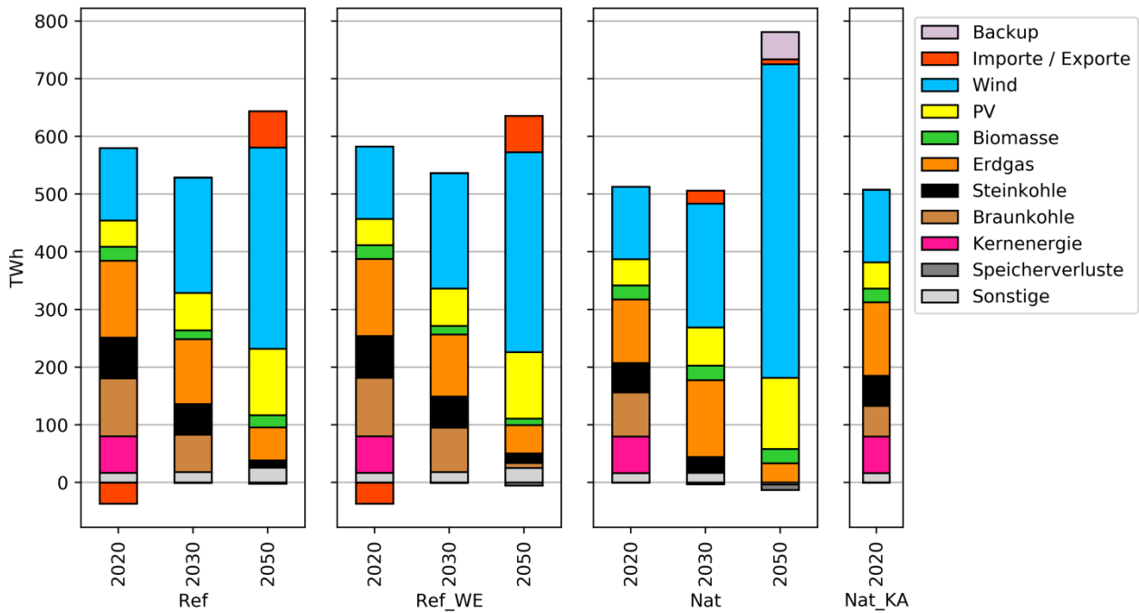
Abbildung 4-17: Erzeugungsmix Strom
