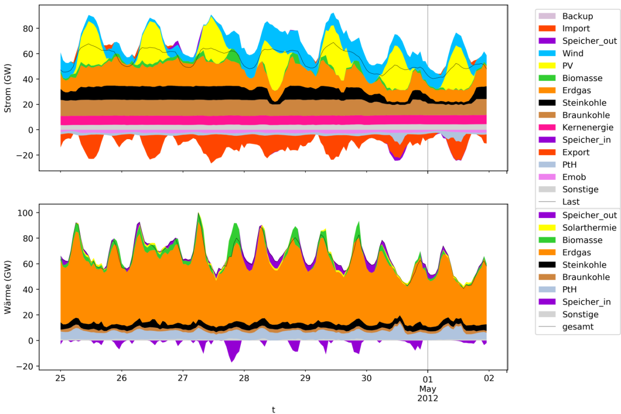
Abbildung 4-21: Strom- und Wärmeerzeugung in stündlicher Auflösung (Aprilwoche, Referenzszenario 2020)
