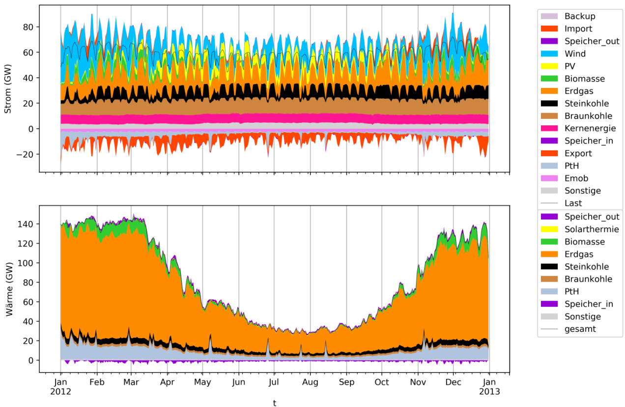
Abbildung 4-23: Strom- und Wärmemix im Jahresgang (Referenzszenario 2020)
