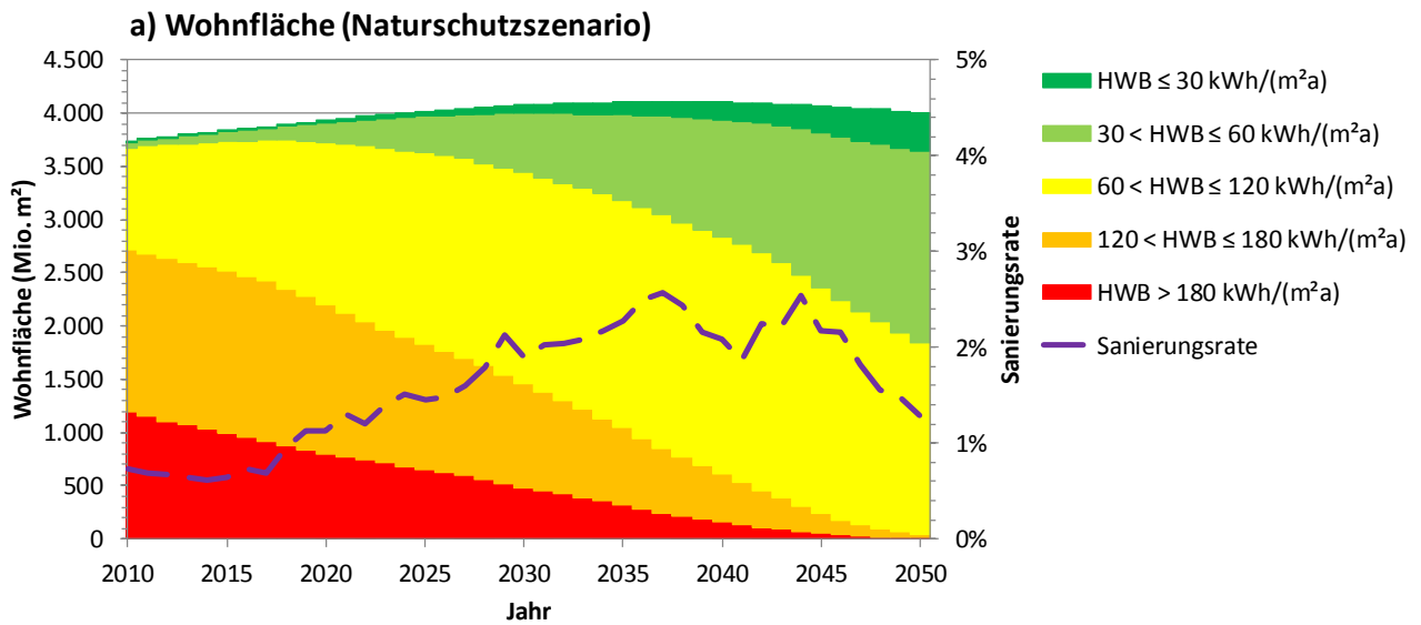
Abbildung 3-4: Sanierungsrate und Wohn-/Nutzflächen im Naturschutzszenario
