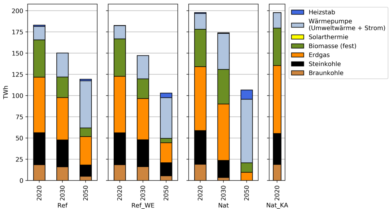
Abbildung 4-11: Erzeugungsmix Fernwärme
