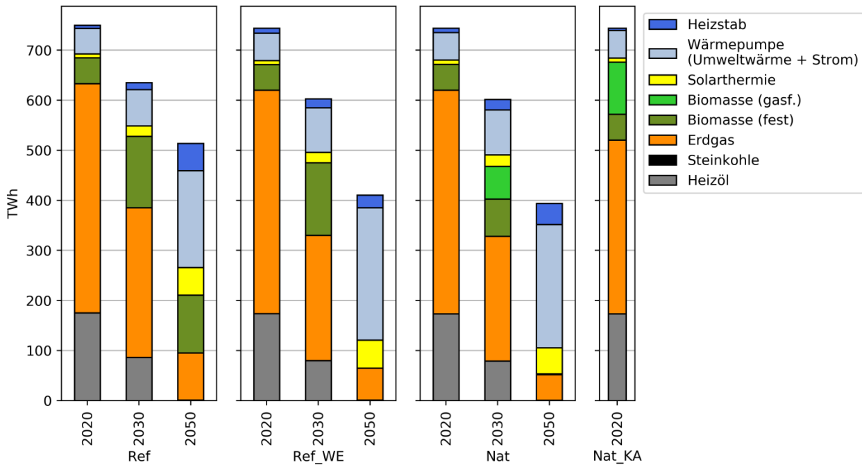
Abbildung 4-9: Erzeugungsmix dezentrale Wärmeversorgung
